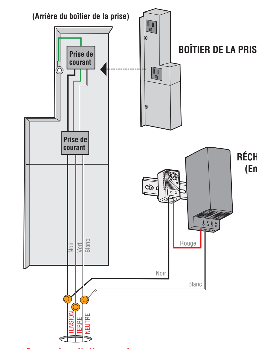
Connexion d'alimentation
